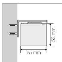
VISTA DI LATO: Attacco a parete con supporto "linguetta U"(OPTIONAL PAG00)
