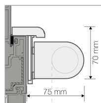
SEZIONE LATERALE MED Profilo su anta
