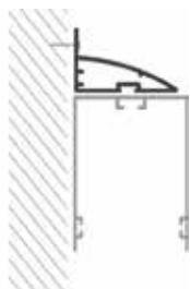
Front Fix aletta esterna 44 x 27 mm
