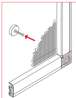
Attacco con angolo magnetico in appoggio su superficie
