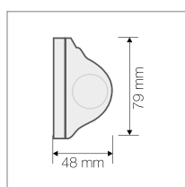
SEZIONE CASSONETTO Attacco su anta con biadesivo
