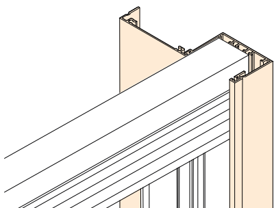
Kit incasso Ghost
