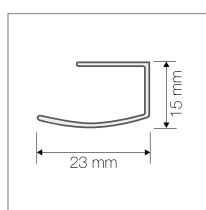
SEZIONE GUIDA LATERALE Attacco su anta con biadesivo
