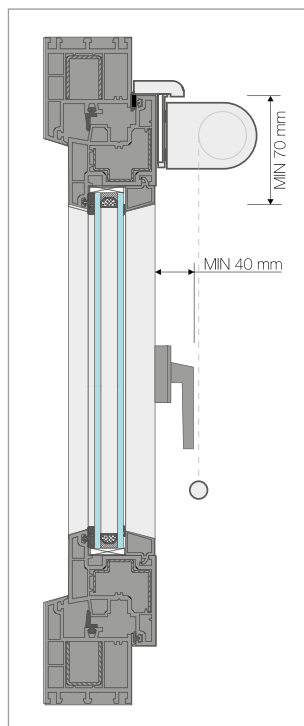
VERIFICA DELLE MISURE VISTA DI LATO - Attacco su anta
