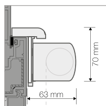
SEZIONE LATERALE MIN Profilo su anta
