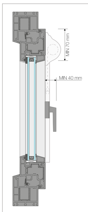
VERIFICA DELLE MISURE VISTA DI LATO - Attacco su anta,
