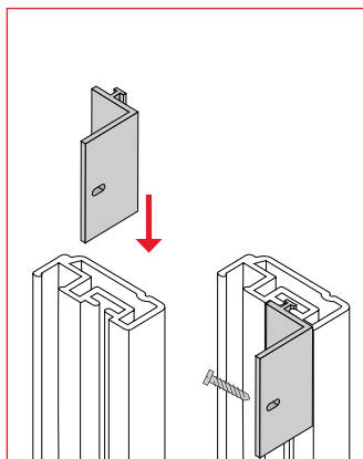
Attacco a muro (interno vano)
