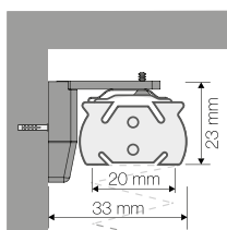
VISTA DI LATO Per comando a maniglia con attacco a parete
