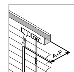
ASTA E PROFILO (A+P) Fermacorda + orientatore = 3,5 cm
